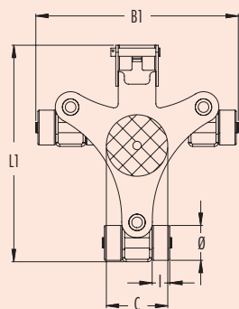
Dessin JKB 1,5 K Schets JKB 1,5 K
