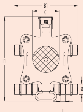
Dessin JKB 6 K Schets JKB 6 K
