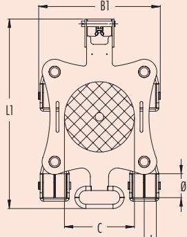
Dessin JKB 3 K Schets JKB 3 K
