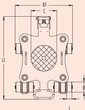
Dessin JKB 4 K Schets JKB 4 K
