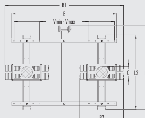
Dessin JTLB 14 K Schets JTLB 14 K
