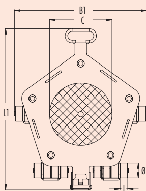
Dessin JKB 7,5 K Schets JKB 7,5 K
